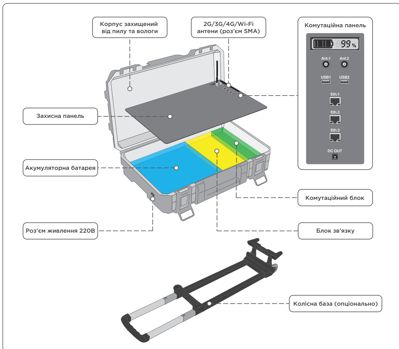
Конструкція пересувного комплексу Pilgrim
